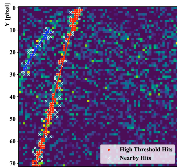
径迹重建结果
