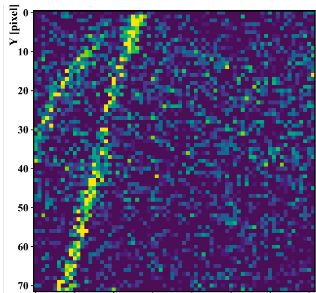
Topmetal II直接测量得到的 电离径迹
