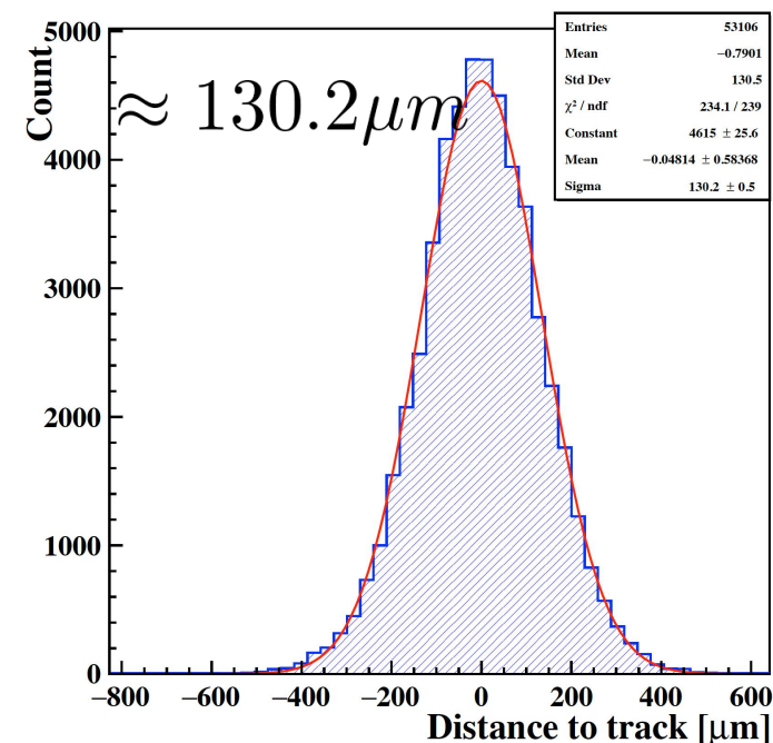
SVD拟合后统计得到的径迹 横向分布
