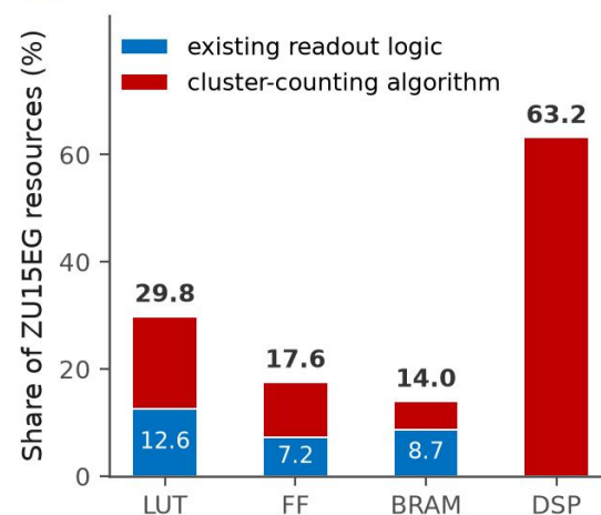
(b) Total utilisation on the ZU15EG
