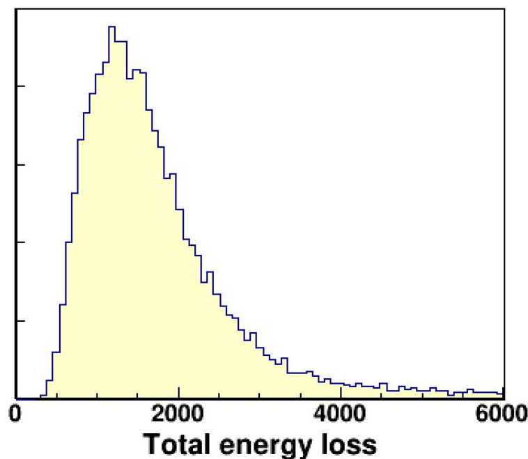
dE/dx : total charge
