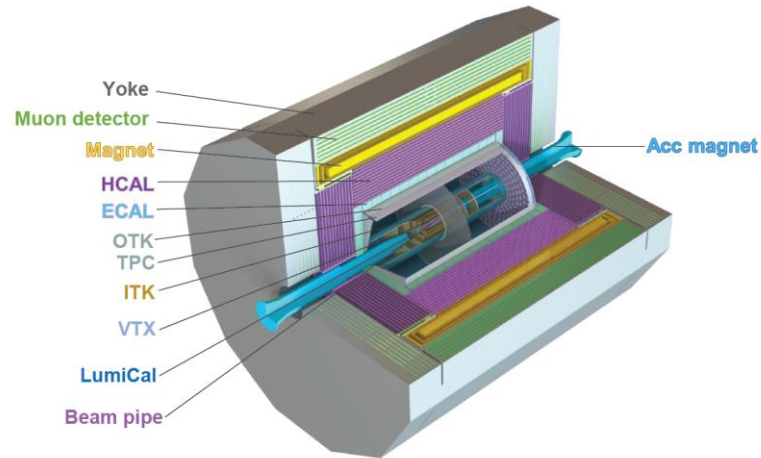
AGORA detector for CEPC
