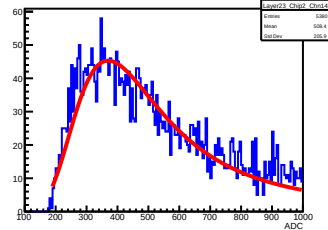
Layer23_Chip2_Chn14
