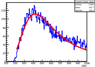
Layer23_Chip2_Chn8
