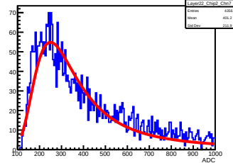
Layer22_Chip2_Chn7
