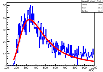
Layer17_Chip2_Chn6
