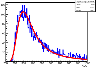
Layer6_Chip2_Chn13
