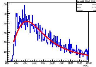
Layer19_Chip2_Chn6
