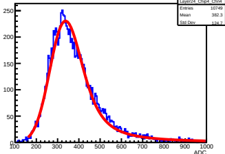
Layer24_Chip4_Chnl4
