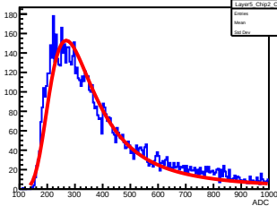
Layer5_Chip2_Chn11
