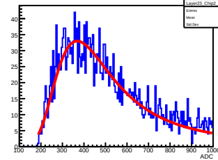
Layer23_Chip2_Chn5
