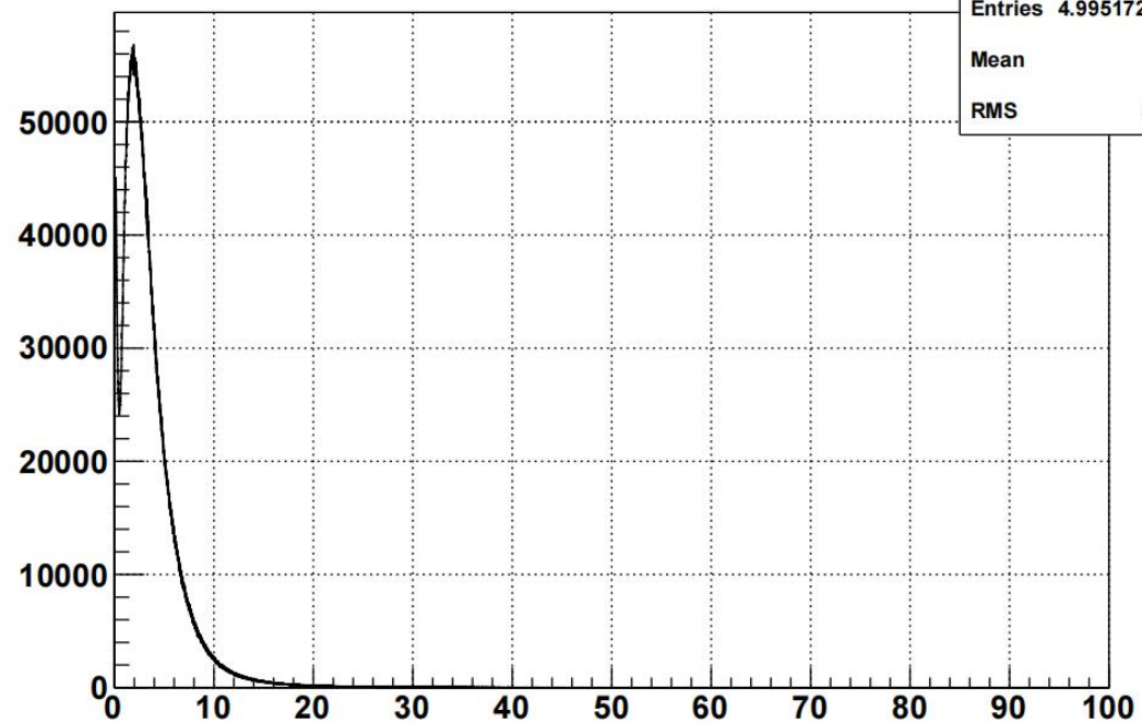
hdca_pi
